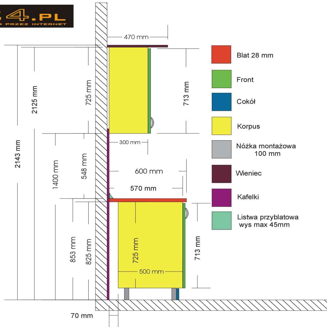
Rysunek poglądowy rozmieszczenia i wymiarów elementów zabudowy kuchennej w wersji standardowej.
